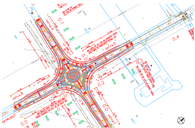
Pôdorys križovatky podľa stavebného projektu.
